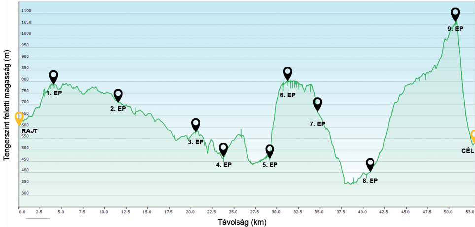
ÚTVONALPROFIL
